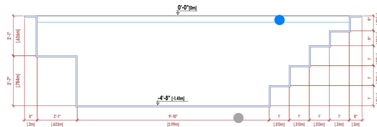
LONGITUDINAL SECTION A-A
