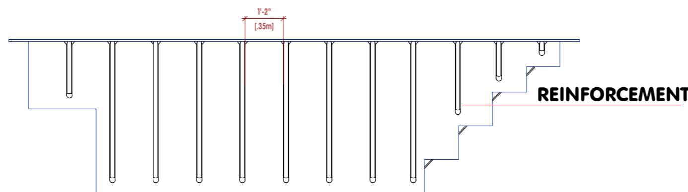
LONGITUDINAL SIDE VIEW C-C
