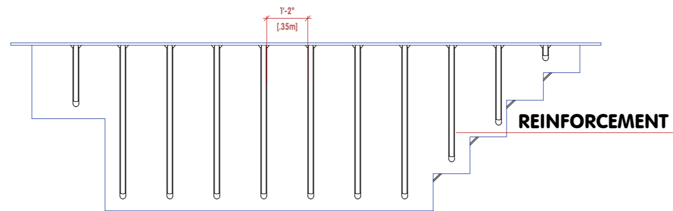
LONGITUDINAL SIDE VIEW C-C
